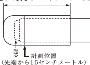
図 竹刀の先革長、先革先端部最小直径値、ちくとう直径値の計測方法
